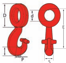
Crochet coulissant
