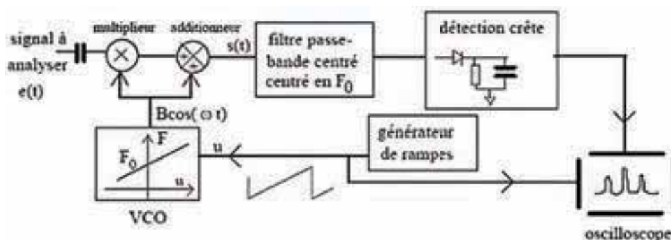
Synoptique d'un analyseur de spectre hétérodyne
