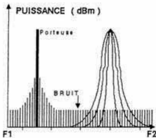
Mesure du bruit avec plusieurs filtres d'analyse
