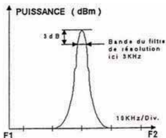
Largeur du filtre d'analyse
