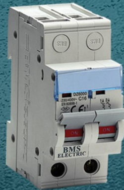
MD2 Mini disjoncteur 10A/16/ 20A/32A
