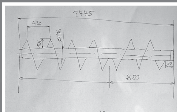
Rozměrový náčrt opotřebovaného dílu
