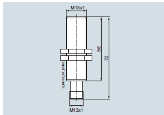
Transmetteur d'impulsions BIS-M18E-Y1X-H1141
