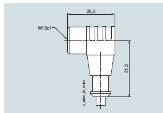
Rundsteckverbinder WWAK4.21-2/P00
