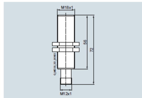
Impulsgeber BL5-M18E-Y1X-H1141
