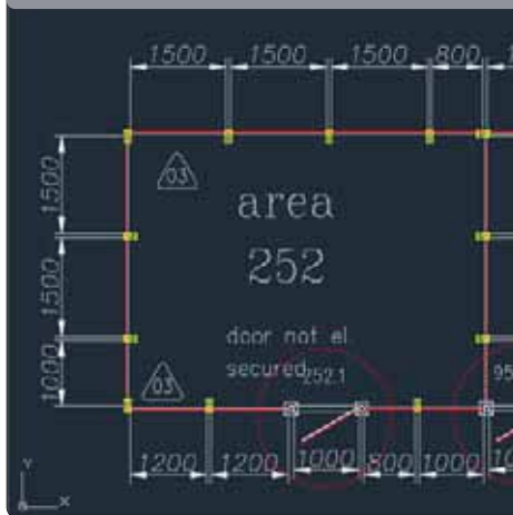
PROGETTAZIONE AUTOCAD
