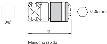
Mandrino rapido
