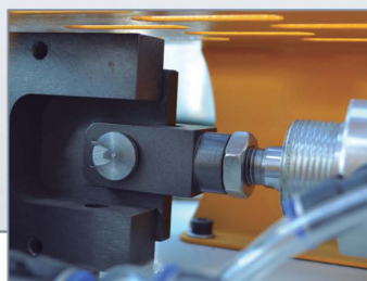
Cizalla de corte neumático Pneumatic cutting shears Guillotine de coupe pneumatique
