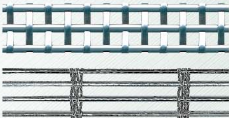
Halbrund-Leinenbindung
