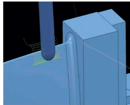
Fräsbahnerzeugung im adaptiven CAM-System
