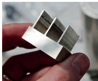
Laserauftragsgeschweißtes Material
