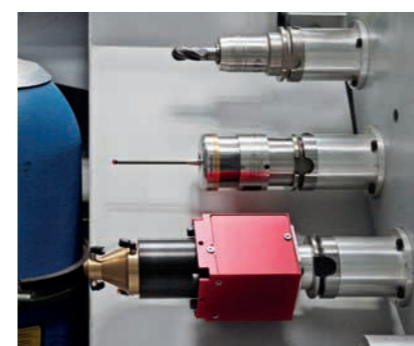
Werkzeug, Messtaster und Laserschweißeinheit im Werkzeugwechsler
