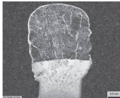
Materialprobe zum Nachweis der optimalen Verbindung des aufgetragenen Materials
