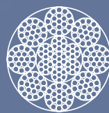
8 x 7+1 x 19
