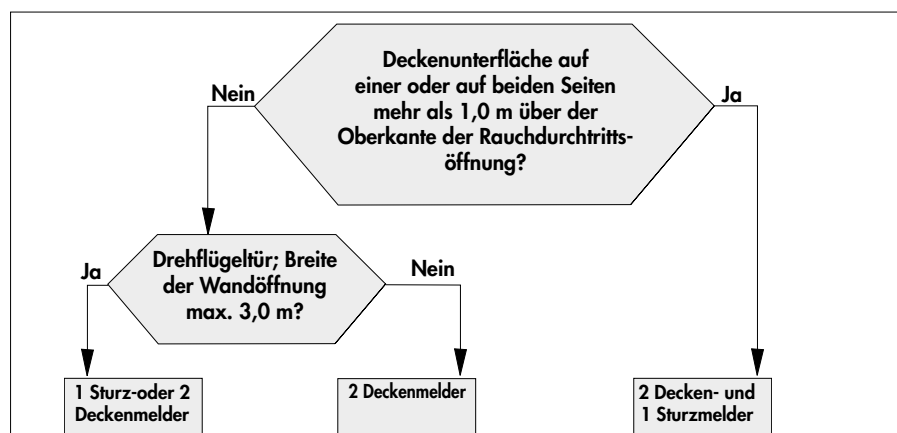
Bild 3: Entscheidungsdiagramm
