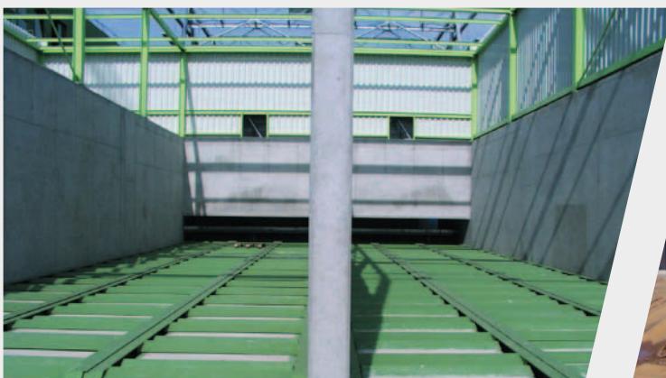
Überfahrbare Schuboden im Bunker eines Biomassekraftwerks
