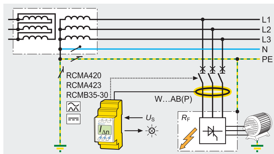
Vigilancia de accionamientos regulados
