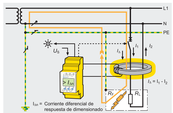
Principio de funcionamiento de un RCM tipo A
