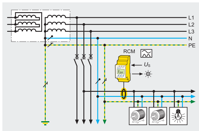
Vigilancia de varios consumidores eléctricos
