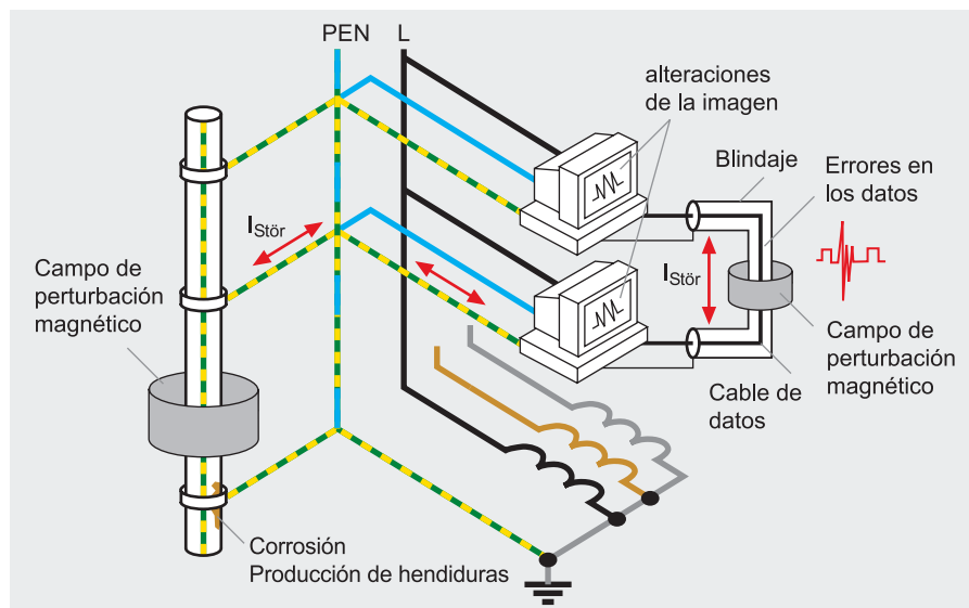
Sistema TN-C no favorable para la compatibilidad electromagnética (4 conductores)
