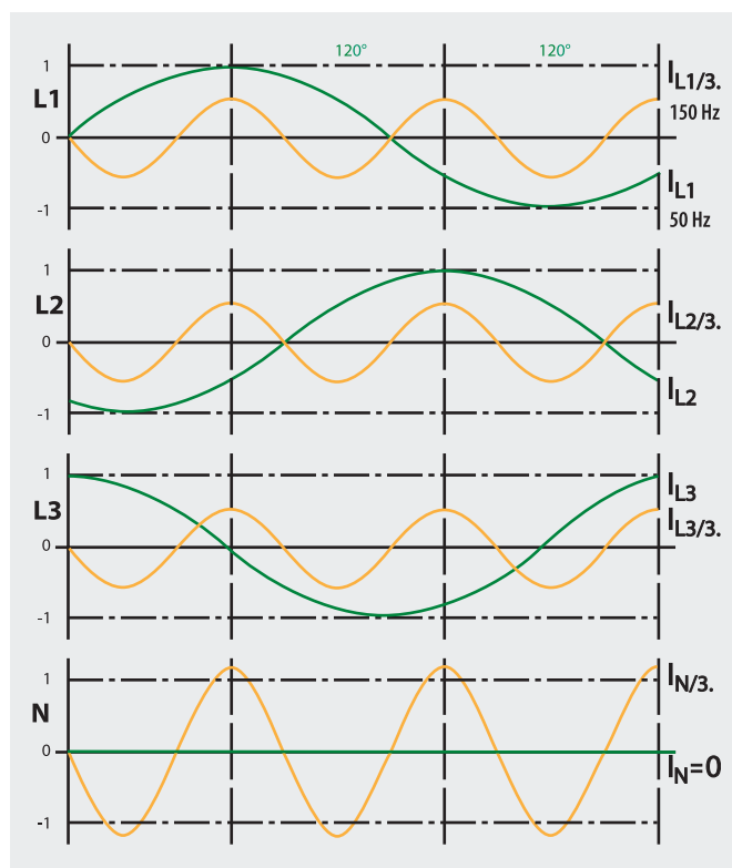
Las corrientes de 150 Hz del conductor de fase se suman en el conductor N
