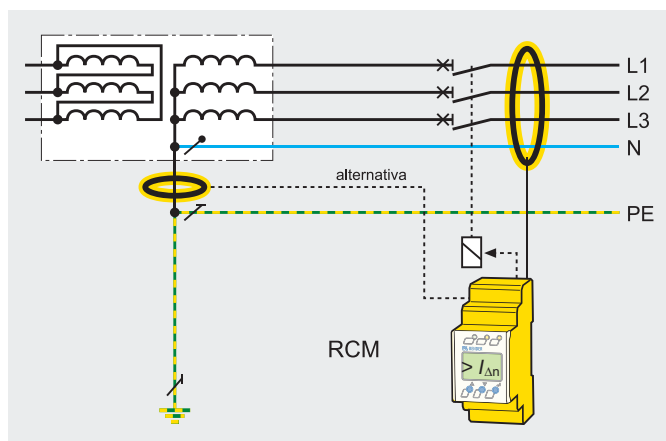
Vigilancia de una alimentación para detectar corrientes de error (Conductor o PE)
