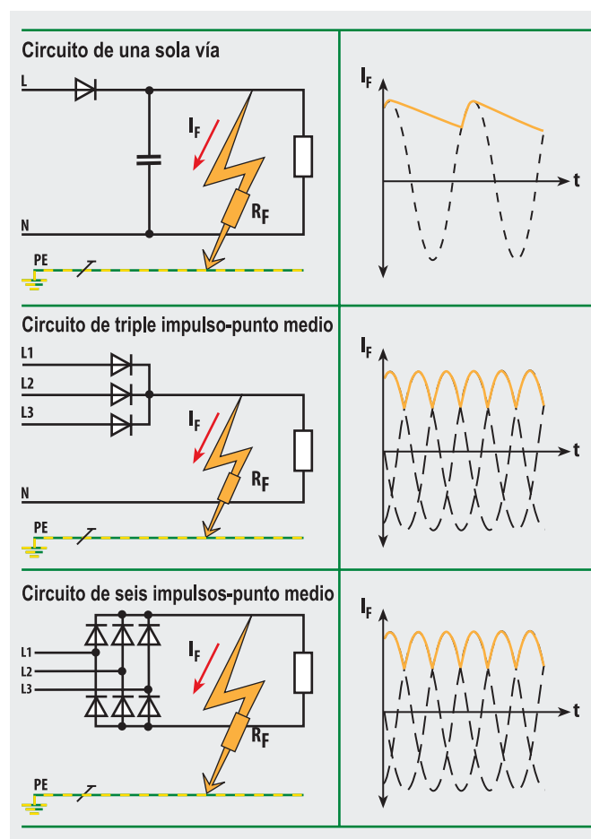
Circuitos rectificadores con corriente continua sin paso por cero
