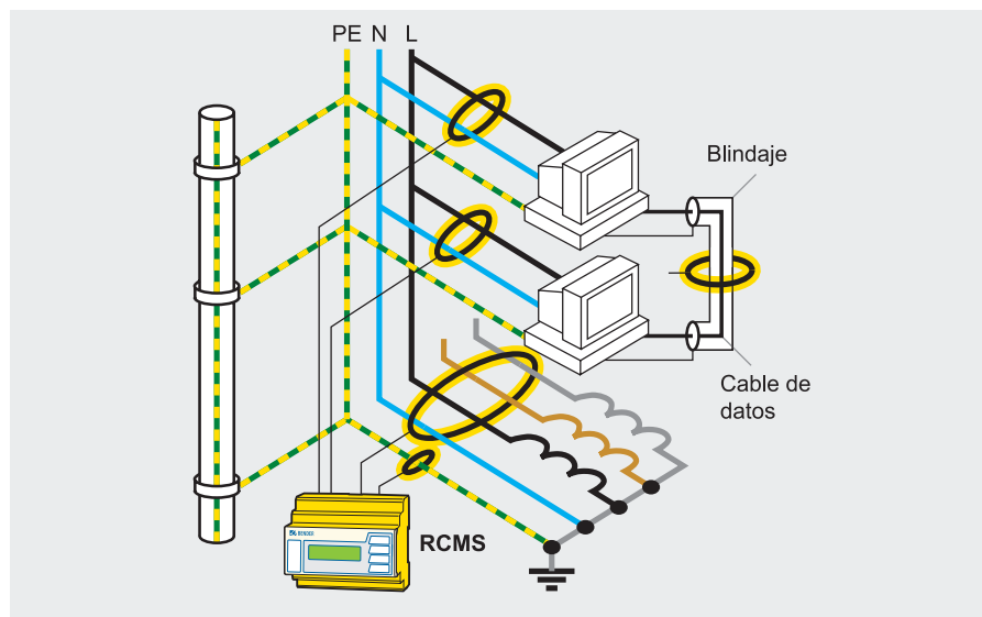
Sistema TN-S ventajoso para la compatibilidad electromagnética (5 conductores) en instalaciones informáticas
