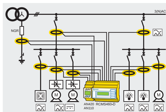
Imagen 2: Detección selectiva de corriente de defecto con RCMS
