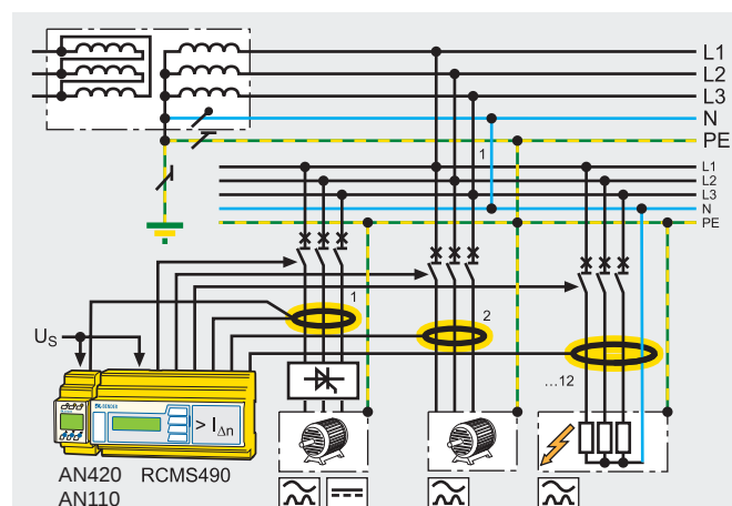
Sistema RCMS490 con función de conmutación por canal de medida
