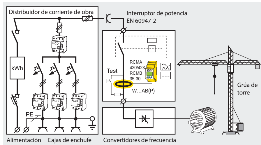
Vigilancia de aparatos de servicio controlados por frecuencia en obra
