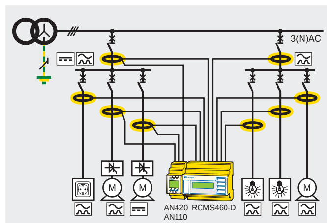
Sistema básico RCMS
