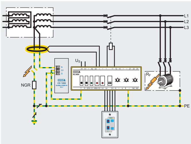
Imagen 3: Vigilancia de fallos a tierra y resistencia de puesta a tierra con RC48N
