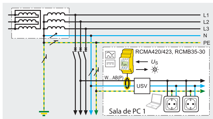
Vigilancia de salas de ordenadores
