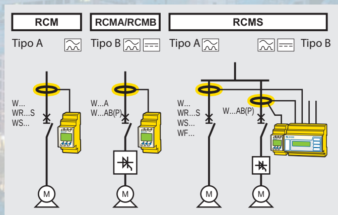
Aplicación de RCM/RCMA/RCMB/RCMS
