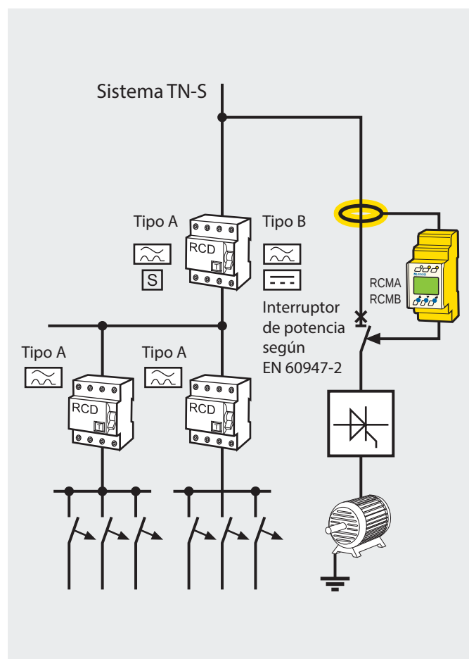
Ejemplo de instalación según DIN EN50178 (VDE 0160): 1998-04
