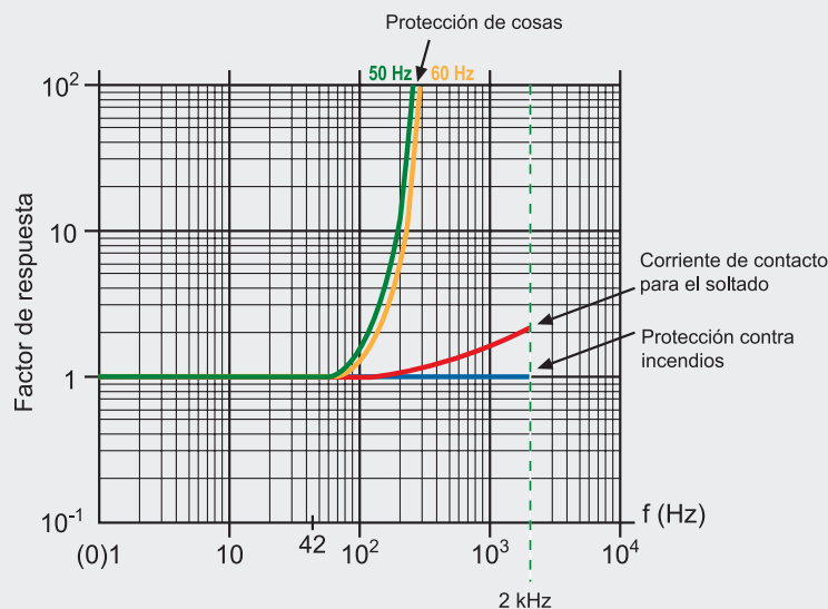
Respuesta en frecuencia según los objetivos de protección
