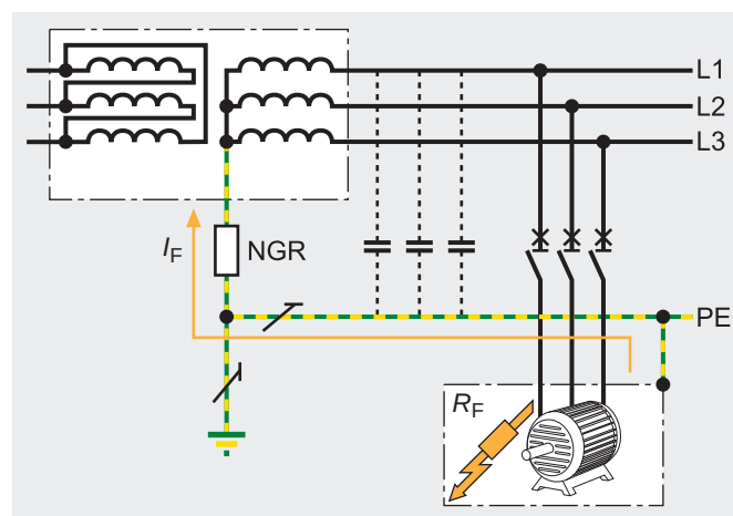
Imagen 1: I_F Corriente de defecto en un fallo fase-tierra
