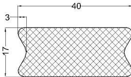
cod:VLC 07-089 material: EPDM 70°Sh
