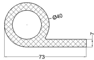
cod:VLC 07-012 material: EPDM 70°Sh
