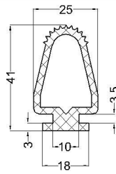
cod:VLC 07-097 material: EPDM 70°Sh
