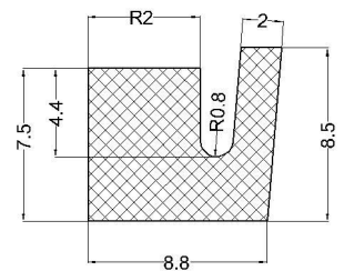
cod:VLC 07-095 material: NBR 60°Sh
