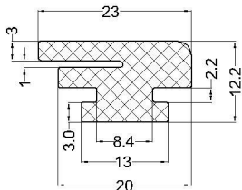
cod:VLC 07-074 material: EPDM 70°Sh
