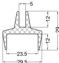
cod:VLC 07-066 material: EPDM 60°Sh
