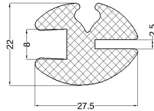
cod:VLC 07-006 material: EPDM 60°Sh
