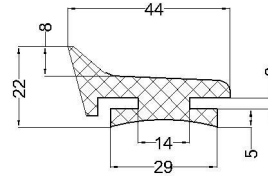
cod:VLC 07-055 material: EPDM 60°Sh
