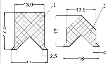
cod:VLC 07-118 material: EPDM 60°Sh
