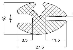
cod:VLC 07-095 material: EPDM 70°Sh
