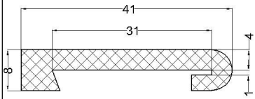
cod:VLC 07-053 material: EPDM 70°Sh
