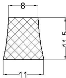
cod:VLC 07-085 material: NBR 80°Sh
