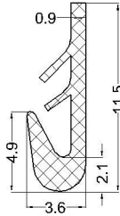
cod:VLC 07-053 material: EPDM 70°Sh
