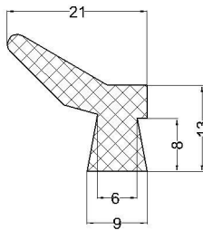
cod:VLC 07-081 material: NBR 60°Sh
