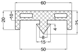
cod:VLC 07-101 material: EPDM 70°Sh
