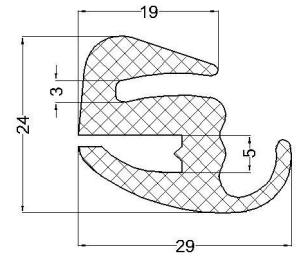
cod:VLC 07-060 material: EPDM 70°Sh
