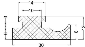
cod:VLC 07-016 material: EPDM 70°Sh
