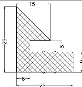
cod:VLC 07-078 material: EPDM 70°Sh
