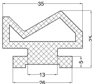
cod:VLC 07-105 material: EPDM 70°Sh
