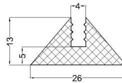
cod:VLC 07-079 material: EPDM 70°Sh
