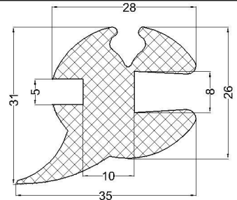
cod:VLC 07-008 material: EPDM 70°Sh
