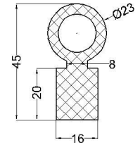
cod:VLC 07-068 material: EPDM 50°Sh
