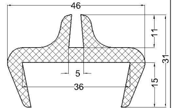
cod:VLC 07-020 material: EPDM 60°Sh
