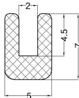
cod:VLC 07-062 material: EPDM 60°Sh
