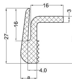
cod:VLC 07-023 material: EPDM 70°Sh
