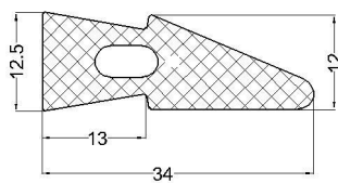
cod:VLC 07-017 material: NBR 70°Sh
