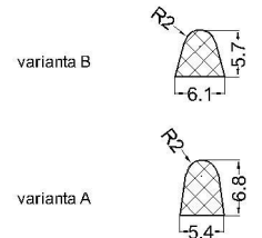
cod:VLC 07-112 material: NBR 70°Sh
