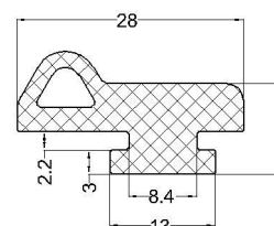
cod:VLC 07-067 material: NBR 70°Sh
