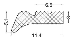
cod:VLC 07-116 material: NBR 70°Sh
