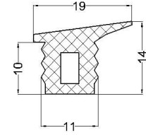
cod:VLC 07-056 material: EPDM 70°Sh
