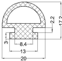
cod:VLC 07-073 material: EPDM 70°Sh
