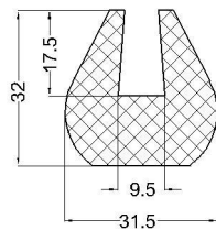
cod:VLC 07-058 material: EPDM 70°Sh
