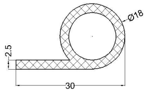
cod:VLC 07-049 material: EPDM 70°Sh
