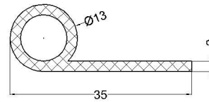
cod:VLC 07-011 material: EPDM 70°Sh
