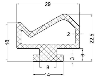
cod:VLC 07-064 material: EPDM 60°Sh
