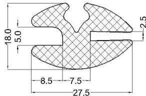
cod:VLC 07-099 material: EPDM 70°Sh
