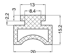
cod:VLC 07-072 material: EPDM 70°Sh
