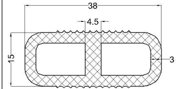
cod:VLC 07-080 material: EPDM 70°Sh
