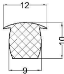
cod:VLC 07-009 material: EPDM 70°Sh
