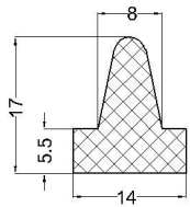
cod:VLC 07-001 material: NBR 70°Sh
