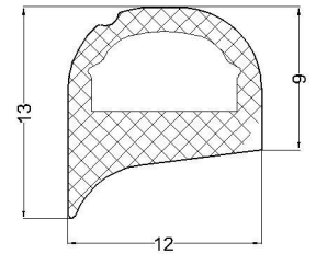
cod:VLC 07-100 material: EPDM 60°Sh
