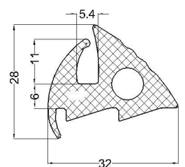
cod:VLC 07-120 material: EPDM 70°Sh
