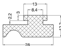
cod:VLC 07-070 material: EPDM 70°Sh
