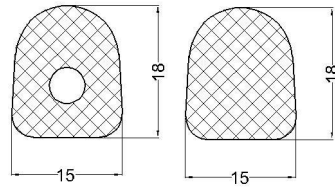
cod:VLC 07-002 material: NBR 60°Sh
