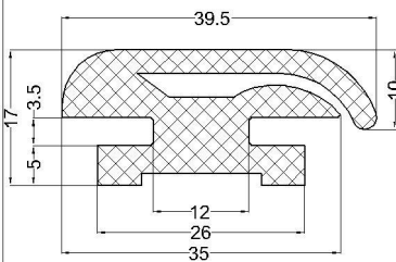
cod:VLC 07-106 material: EPDM 70°Sh
