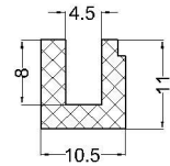
cod:VLC 07-104 material: NBR 50
