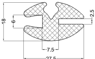
cod:VLC 07-018 material: EPDM 70°Sh
