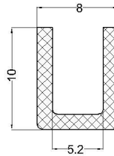
cod:VLC 07-087 material: EPDM 70°Sh
