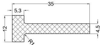
cod:VLC 07-057 material: EPDM 70°Sh
