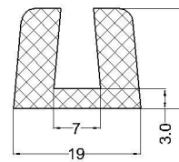
cod:VLC 07-019 material: EPDM 70°Sh
