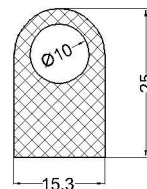
cod:VLC 07-114 material: EPDM 60°Sh
