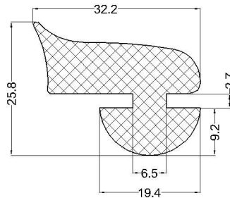
cod:VLC 07-007 material: EPDM 70°Sh
