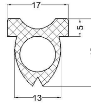
cod:VLC 07-003 material: NBR 60°Sh
