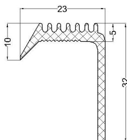
cod:VLC 07-021 material: EPDM 60°Sh
