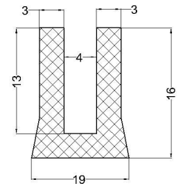
cod:VLC 07-088 material: NBR 60°Sh
