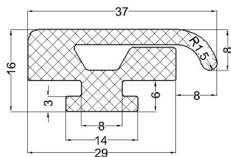
cod:VLC 07-065 material: EPDM 60°Sh
