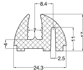
cod:VLC 07-119 material: EPDM 70°Sh
