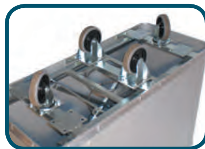
Possibilité de roues en position losange ou en carré
