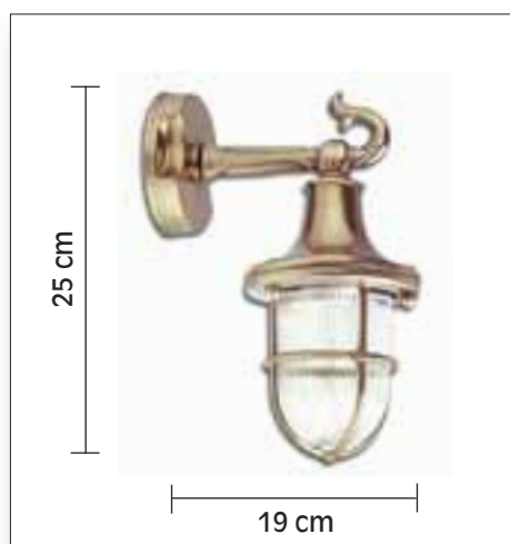
WALL LIGHT 441 ΜΠΡΟΝΖΕ / BRASS
