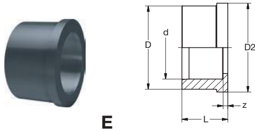
621.60.01 PVC-U Verschraubung Einlegteil grau PVC-U Union Insert-part grey
