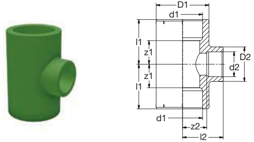
G 8130 red PP-R T-Stück 90° red grün PP-R Tee 90° red green
