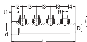
G 8241gB PP-RCT-RG Verteiler AG-keg kaskadierbar grün PP-RCT-Bronze Manifold male-thread-con cascable green
