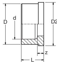
G 8060B PP-RCT Verschraubung Einlegenteil grün PP-RCT Union Insert-part green
