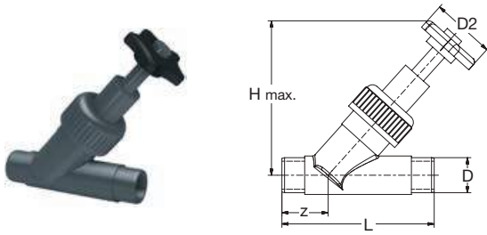
621.300.000 PVC-U Ventil Schrägsitz Runddichtring-PB grau PVC-U Valve angle-seat O-Ring-gasket-PB grey
