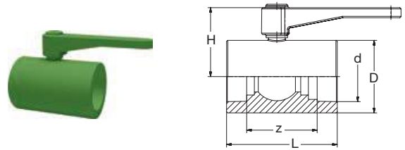
G 8850 PP-R Kugelhahn grün PP-R Ball valve green
