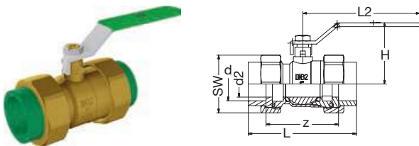
PP-RCT Kugelhahn-Ms verschraubt Runddichtring-EPDM grün PP-RCT Ball valve Brass with union-nuts O-Ring-gasket-EPDM green
