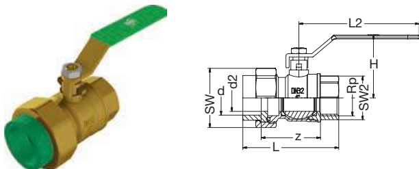
PP-RCT Ü-Kugelhahn-Ms IG-zyl verschraubt Runddichtring-EPDM grün PP-RCT Transition-Ball valve Brass female-thread-cyl with union-nuts O-Ring-gasket-EPDM green
