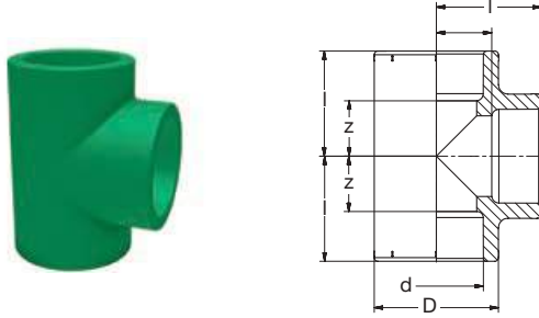
G 8130B PP-RCT T-Stück 90° grün PP-RCT Tee 90° green
