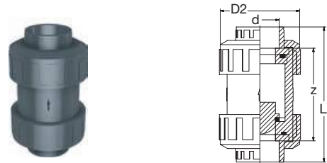
21.10.140 PVC-U Ventil Fuß Runddichtring-EPDM grau PVC-U Valve foot O-Ring-gasket-EPDM grey
