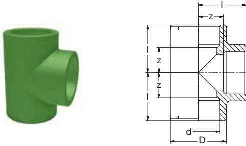
G 8130 PP-R T-Stück 90° grün PP-R Tee 90° green
