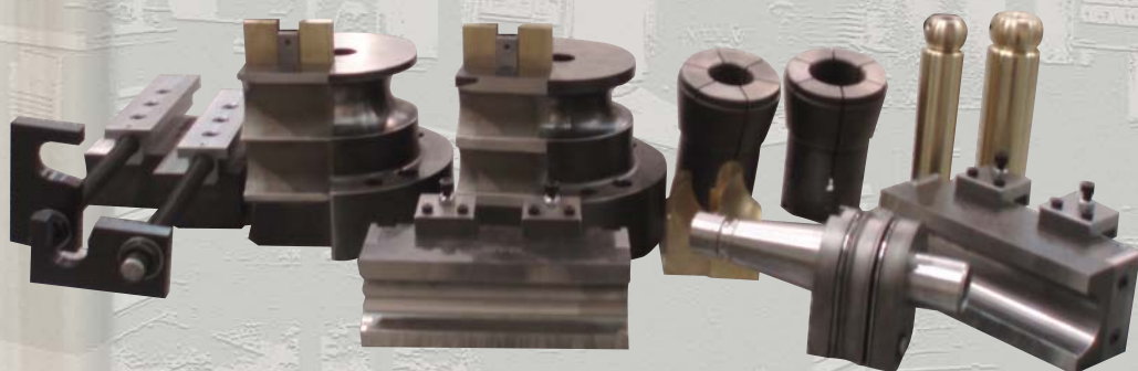
Matrices de dos alturas, pinzas, mandrinos y carriles.
