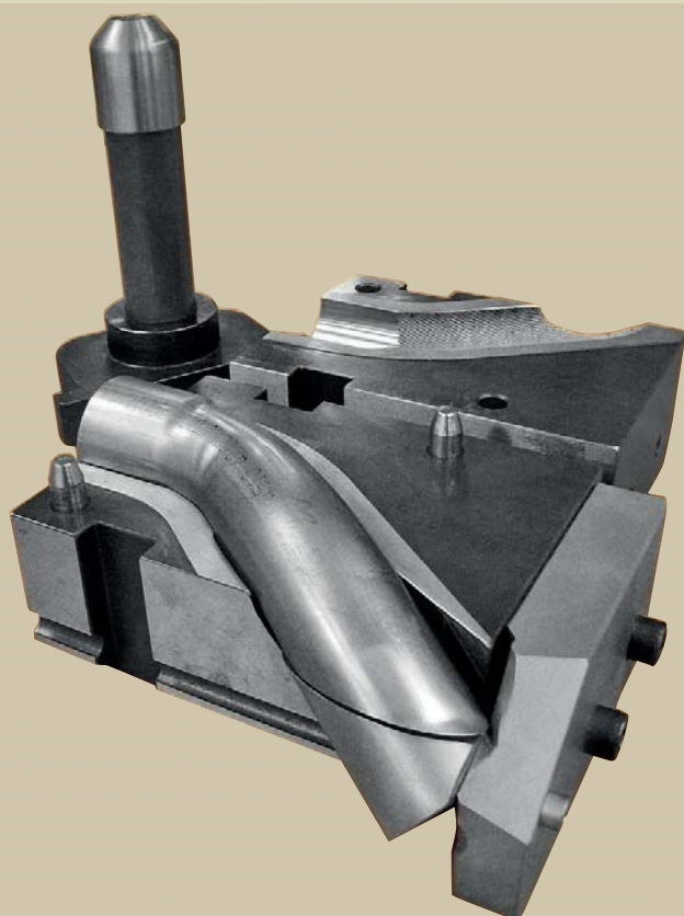
Cunas para el ensanchado en extremos de tubo
