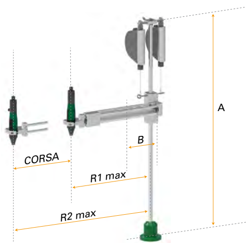
Estensione laterale fino a mm 760
