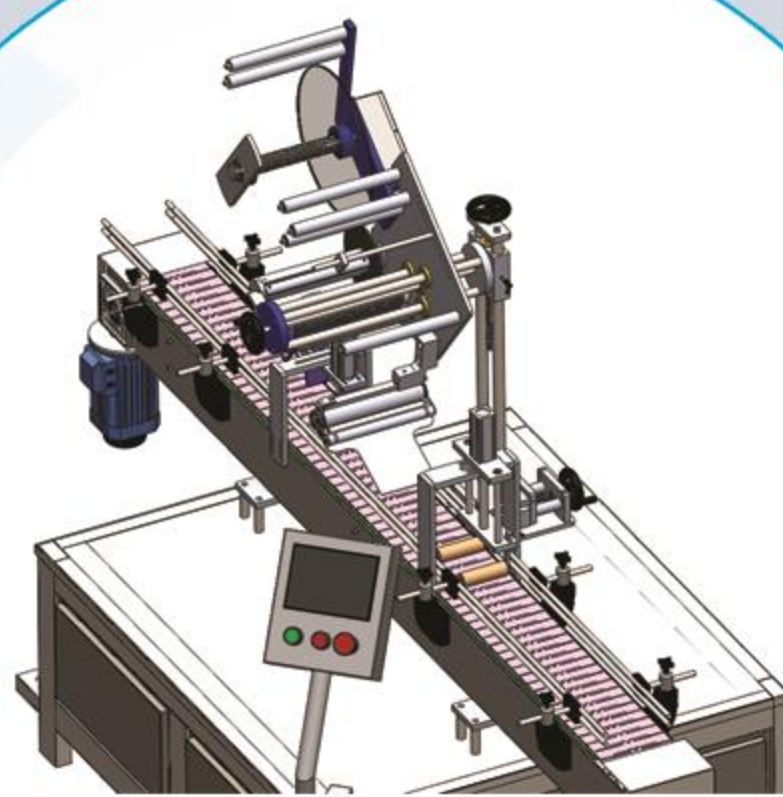
Etiqueteuse automatique face superieure
