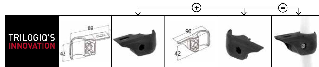
GT-H90A BLACK + GT-H90B BLACK PLATTENHALTER (Teil A) - 45 g PLATTENHALTER (Teil B) - 38 g
