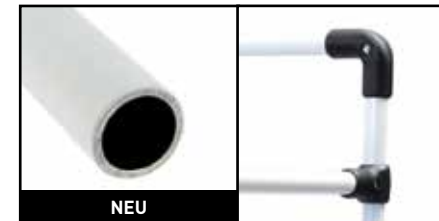
BESCHICHTET - WEIß KOMPATIBEL MIT LEANTEK classic 2MM WANDSTÄRKE, Ø28.6MM, 4000MM LÄNGE - Art.Nr. T2-400 AW
