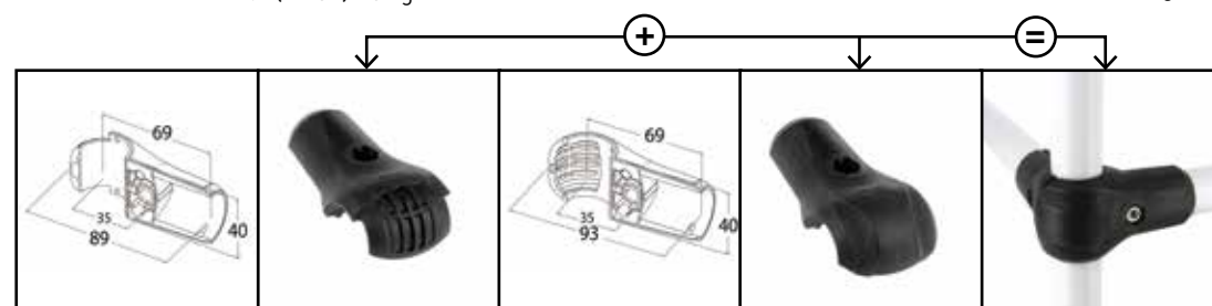
GT-C1 BLACK + GT-C2 BLACK WINKELVERBINDER 270° AUßEN [Teil 1] - 47 g [Teil 2] - 46 g
