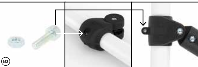
S14W Verstärkter Halt SCHRAUBE UND MUTTER ZUR BEFESTIGUNG VON F-F UND GT-F
