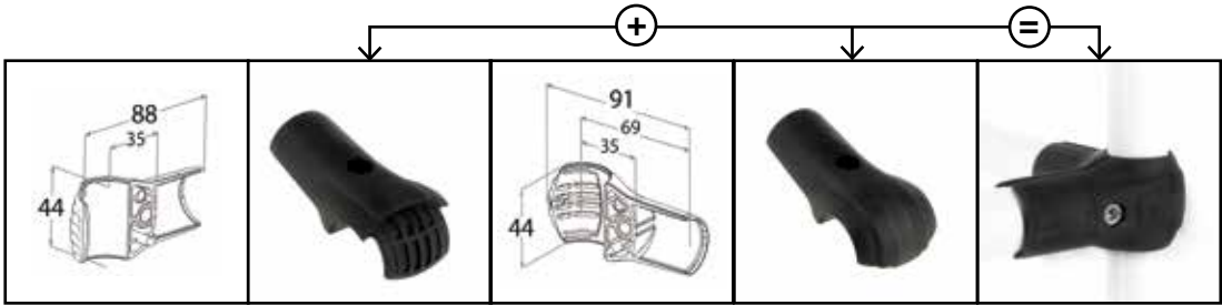
F-C1 BLACK + F-C2 BLACK WINKELVERBINDER 270° [Teil 1] - 34 g WINKELVERBINDER 270° [Teil 2] - 33 g
