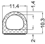
cod: VLC 07-269 material: EPDM buretos
