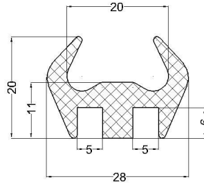
cod: VLC 07-175 material: EPDM 70°Sh
