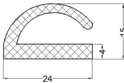
cod: VLC 07-177 material: EPDM 70°Sh
