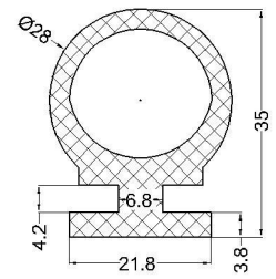
cod:VLC 07-196 material: EPDM 70°Sh
