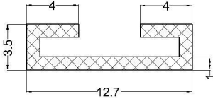
cod:VLC 07-197 material: EPDM 70°Sh
