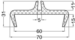
cod:VLC 07-126 material: EPDM 60°Sh
