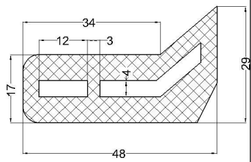
cod: VLC 07-184 material: EPDM 70°Sh
