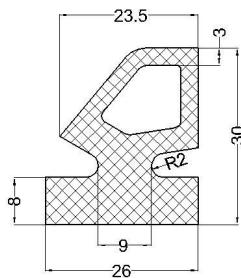
cod: VLC 07-229 material: EPDM 50°Sh
