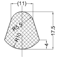
cod: VLC 07-268 material: cauciu alimentar 70°Sh
