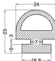
cod: VLC 07-239 material: EPDM 70°Sh
