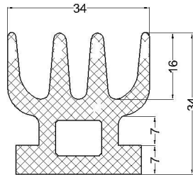
cod: VLC 07-230 material: EPDM 50°Sh
