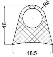
cod: VLC 07-217 material: cauciu siliconic 50°Sh
