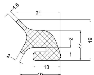
cod: VLC 07-188 material: cauciuc alimentar 60°Sh
