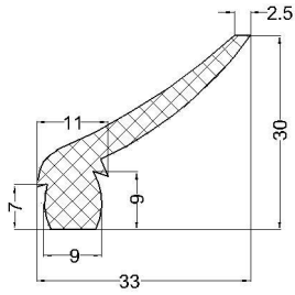
cod:VLC 07-129 material: EPDM 70°Sh
