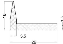
cod:VLC 07-130 material: EPDM 70°Sh
