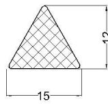
cod: VLC 07-169 material: EPDM 70°Sh
