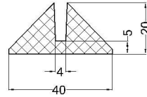
cod:VLC 07-123 material: SBR 70°Sh
