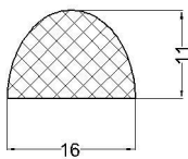
cod:VLC 07-137 material: EPDM 70°Sh
