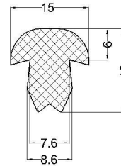
cod: VLC 07-267 material: NBR 70°Sh
