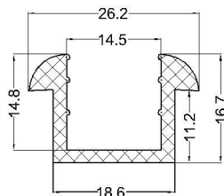
cod: VLC 07-181 material: EPDM 70°Sh
