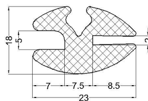
cod: VLC 07-187 material: EPDM 70°Sh
