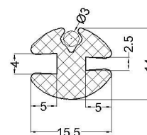
cod:VLC 07-211 material: EPDM 70°Sh
