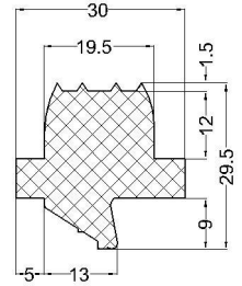
cod:VLC 07-200 material: EPDM 60°Sh
