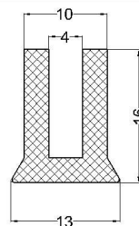
cod: VLC 07-234 material: H 60°Sh
