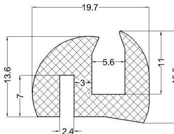
cod: VLC 07-183 material: EPDM 70°Sh
