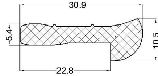
cod: VLC 07-174 material: EPDM 70°Sh
