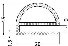
cod:VLC 07-213 material: EPDM 70°Sh
