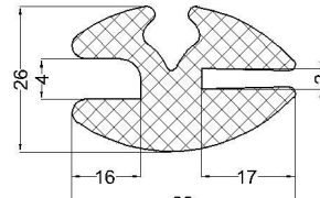
cod: VLC 07-191 material: EPDM 70°Sh
