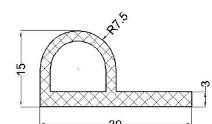
cod: VLC 07-192 material: NBR 70°Sh
