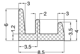
cod:VLC 07-144 material: EPDM 70°Sh
