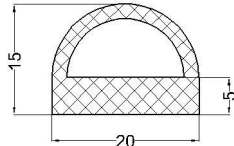
cod:VLC 07-198 material: EPDM 70°Sh
