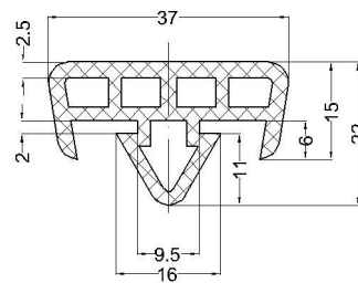
cod: VLC 07-186 material: EPDM 70°Sh
