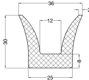
cod:VLC 07-203 material: EPDM 70°Sh
