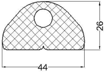
cod:VLC 07-125 material: EPDM buretos
