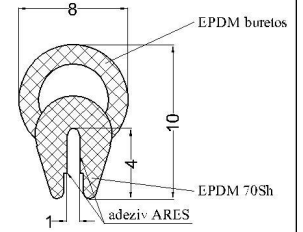
cod: VLC 07-224 material: EPDM 70°Sh
