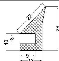
cod: VLC 07-236 material: H 45°Sh
