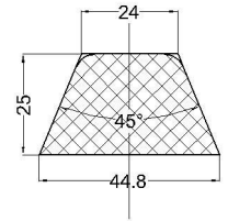
cod:VLC 07-128 material: NBR 80°Sh
