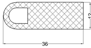
cod:VLC 07-134 material: EPDM 70°Sh
