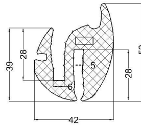
cod: VLC 07-171 material: EPDM 70°Sh
