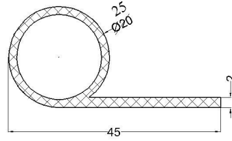
cod:VLC 07-131 material: EPDM 70°Sh
