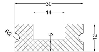
cod:VLC 07-204 material: EPDM 70°Sh
