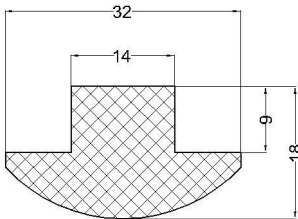
cod:VLC 07-201 material: EPDM 60°Sh
