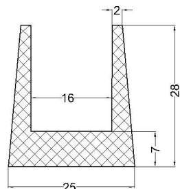
cod: VLC 07-185 material: EPDM 70°Sh
