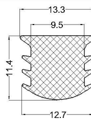
cod: VLC 07-231 material: EPDM buretos
