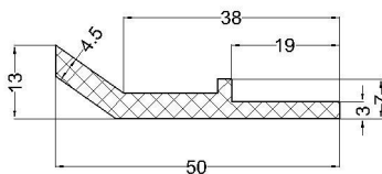
cod:VLC 07-210 material: EPDM buretos
