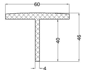
cod:VLC 07-140 material: EPDM 70°Sh
