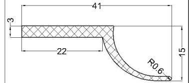
cod: VLC 07-176 material: EPDM 70°Sh
