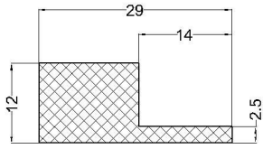
cod: VLC 07-265 material: H 40°Sh
