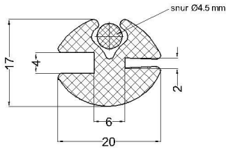
cod: VLC 07-225 material: EPDM 60°Sh
