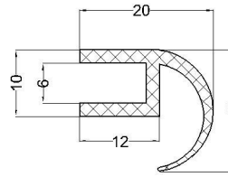
cod:VLC 07-135 material: EPDM 70°Sh
