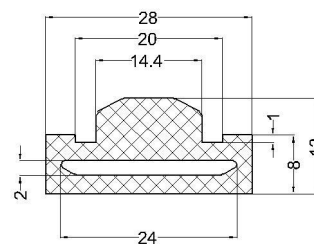
cod: VLC 07-190 material: EPDM 60°Sh
