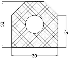
cod:VLC 07-205 material: EPDM 50°Sh
