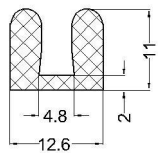
cod: VLC 07-178 material: EPDM 70°Sh
