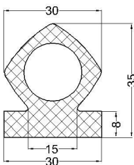
cod:VLC 07-209 material: EPDM buretos
