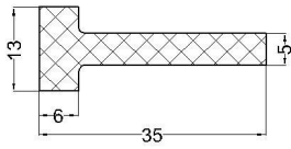
cod: VLC 07-266 material: EPDM 70°Sh
