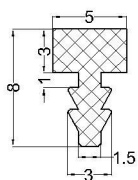
cod: VLC 07-189 material: cauciuc alimentar 70°Sh
