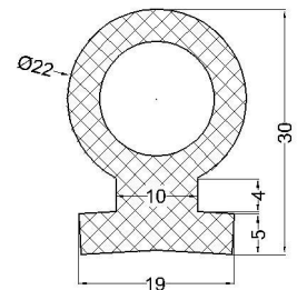
cod: VLC 07-180 material: EPDM 70°Sh
