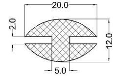
cod: VLC 07-220 material: EPDM 70°Sh
