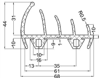
cod:VLC 07-207 material: EPDM 70°Sh
