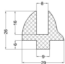
cod:VLC 07-212 material: EPDM 70°Sh
