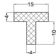
cod:VLC 07-208 material: cauciuc alimentar 60°Sh
