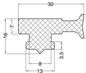
cod:VLC 07-139 material: EPDM 70°Sh
