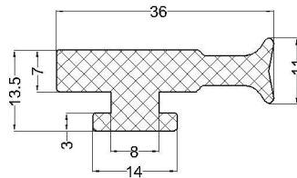
cod:VLC 07-138 material: EPDM 70°Sh
