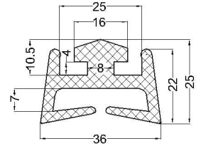
cod:VLC 07-132 material: EPDM 70°Sh
