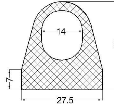
cod:VLC 07-127 material: EPDM 70°Sh
