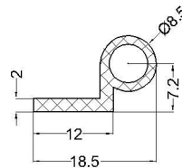
cod: VLC 07-179 material: EPDM 70°Sh
