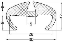
cod:VLC 07-133 material: EPDM 70°Sh
