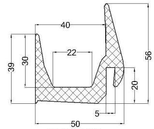
cod: VLC 07-172 material: EPDM 70°Sh
