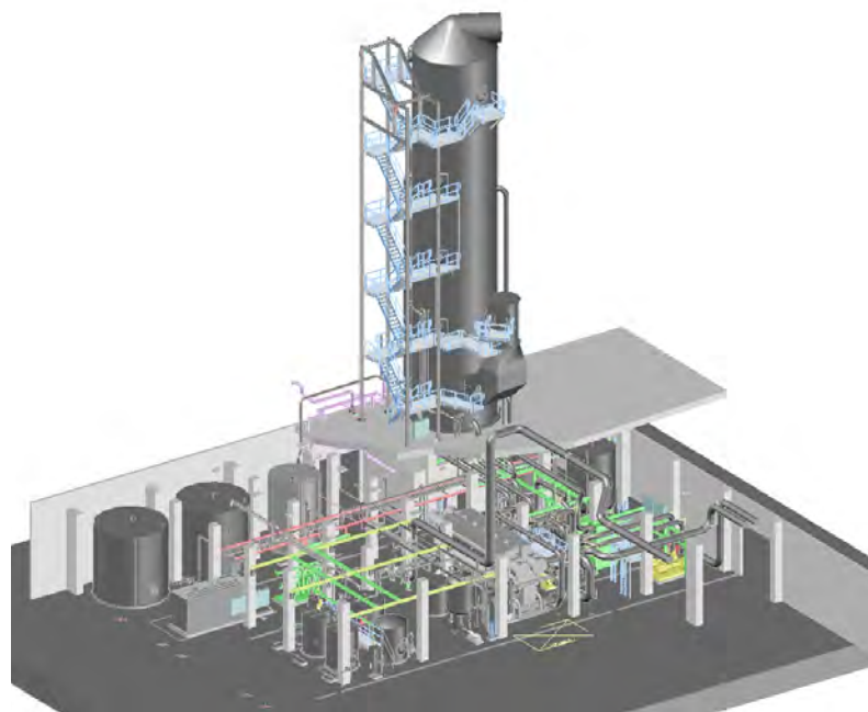
Götaverken Miljö's delivery to Filborna, Helsingborg.
