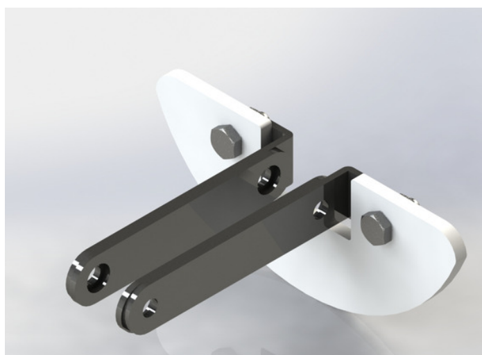
Pala semicircular de polietileno
